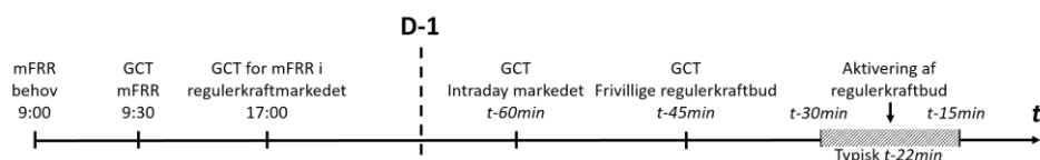
FIGUR 3 | TIDSLINJE FOR MFRR-, REGULERKRAFT- OG INTRADAYMARKEDET TIL DRIFTSTIMEN 'T'
