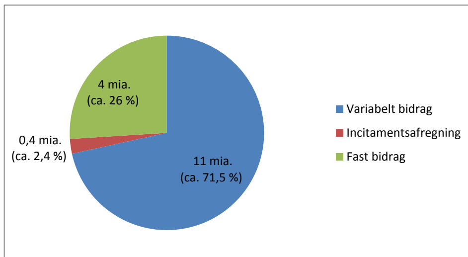
FIGUR 1 | FORDELINGEN AF FJERNVARMEFORSYNINGERNES INDTÆGTER PÅ FASTE BIDRAG, VARIABLE BIDRAG OG INCITAMENTSAFREGNING, 2014/2015.
