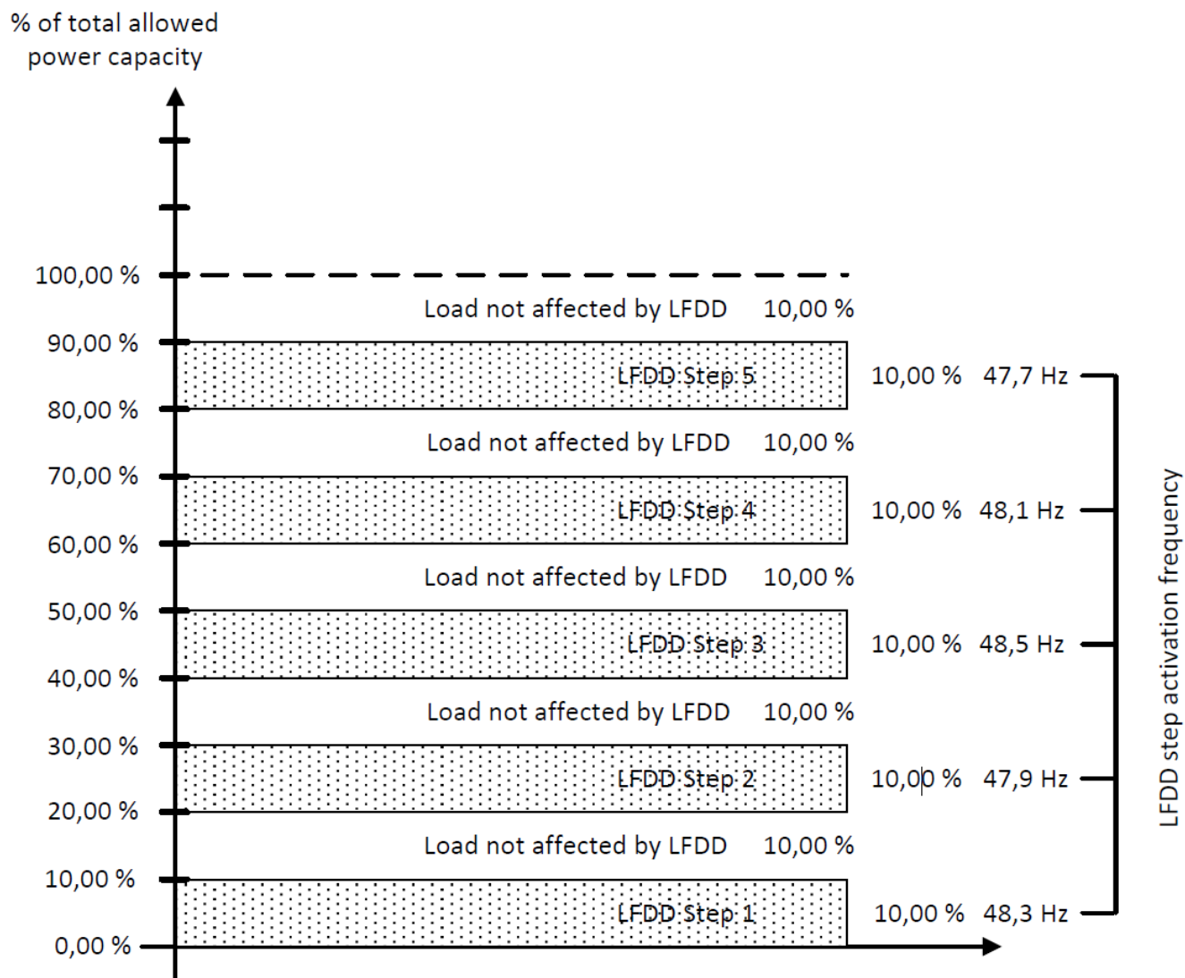
Figur 2: Automatisk LFDD design for kategori 4 - Forbrugsanlæg - Norden
